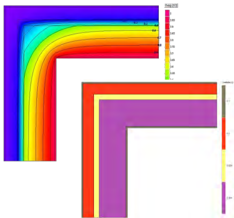
Doppia parete con tramezza esterna
