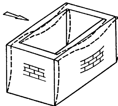
b) con cordolo e con solaio deformabile
