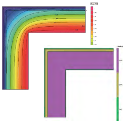
Monostrato con cappotto
