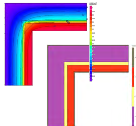
Doppia parete con tramezza interna
